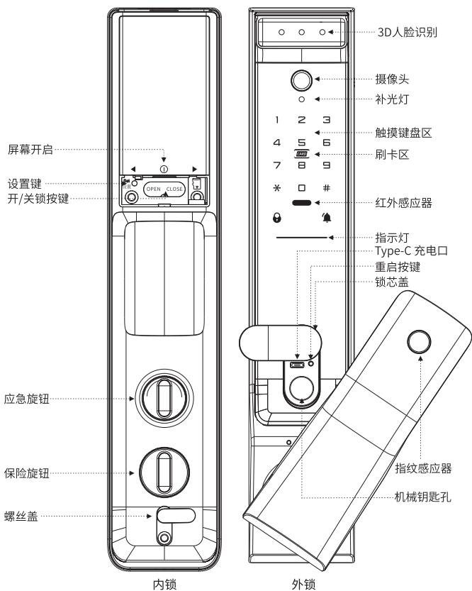
Q3F产品功能图
