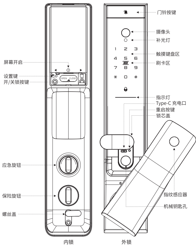
Q3C产品功能图
