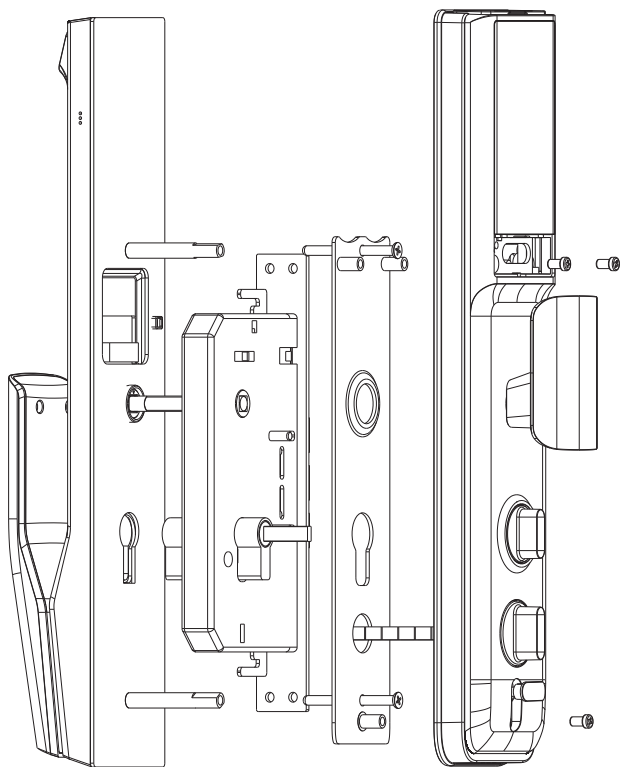
安装示意图
